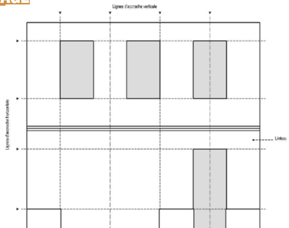
Points d'accroche et lignes de composition des portes cochères ou des portes de garage modernes dans une travée latérale.
