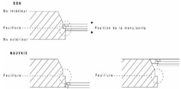
Positionnement des menuiseries nouvelles dans un mur épais ancien.
