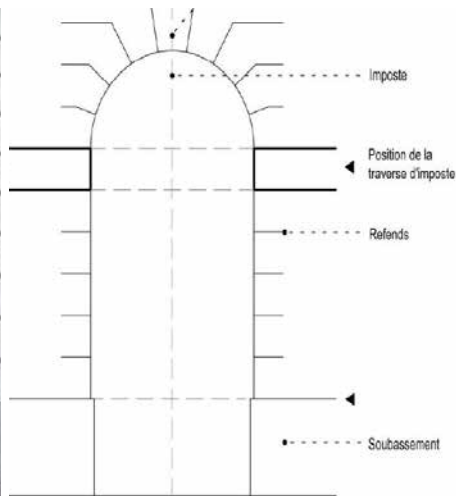
Points d'accroche et lignes de composition des portes d'entrée
